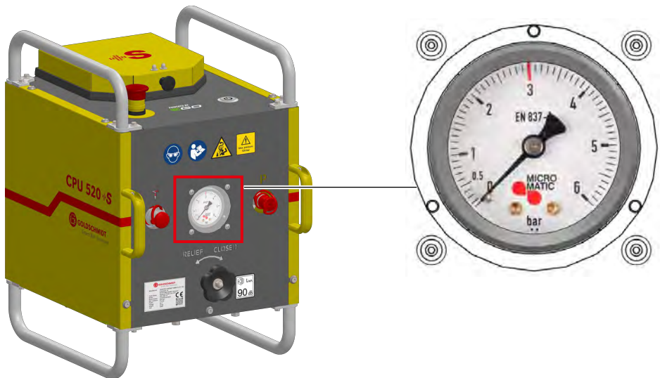
Fig. 2-3 Manomètre haute pression
