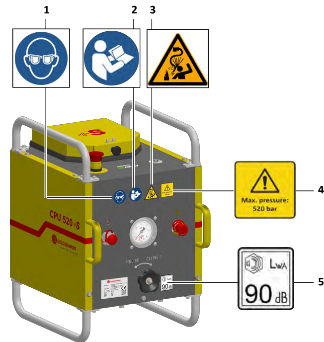
Fig. 2-4 Marquage de sécurité (face avant)
