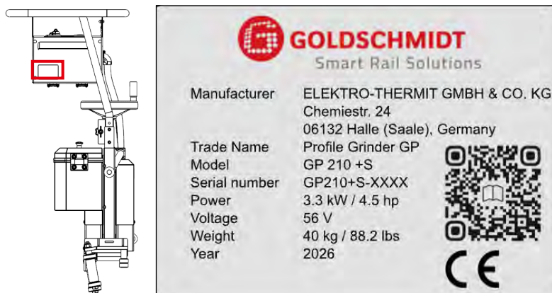
Abb. 2-2 Typenschild
