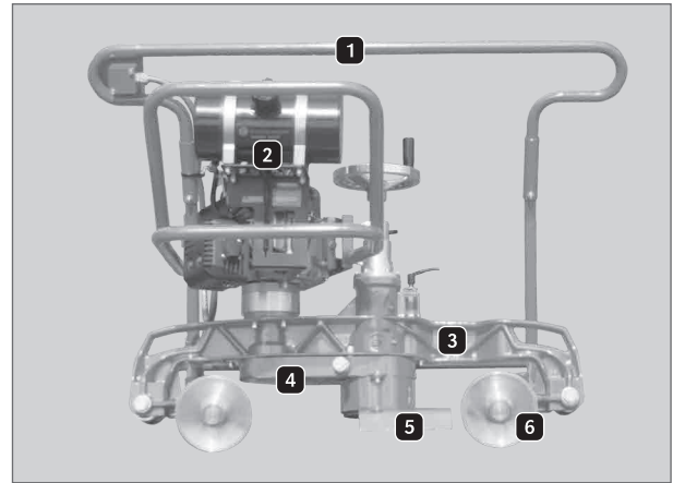
Illustration 10 : Conception globale 1
