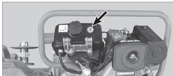
Illustration 5 : Emplacement de montage des panneaux de sécurité 2 GP 4000 D
