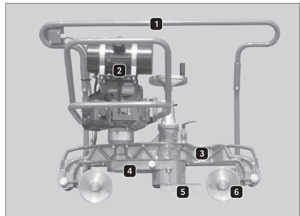
Abbildung 10: Gesamtaufbau 1
