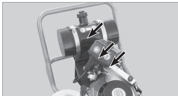
Illustration 7 : Emplacement de montage des panneaux de sécurité 2 GP 4000 P
