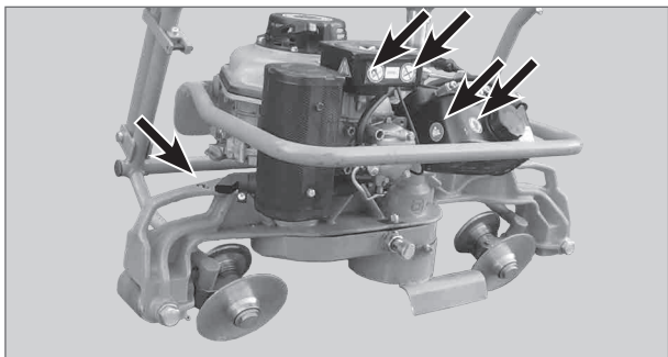
Illustration 4 : Emplacement de montage des panneaux de sécurité 1 GP 4000 D
