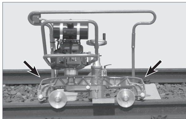
Illustration 11 : Dispositifs porteurs
